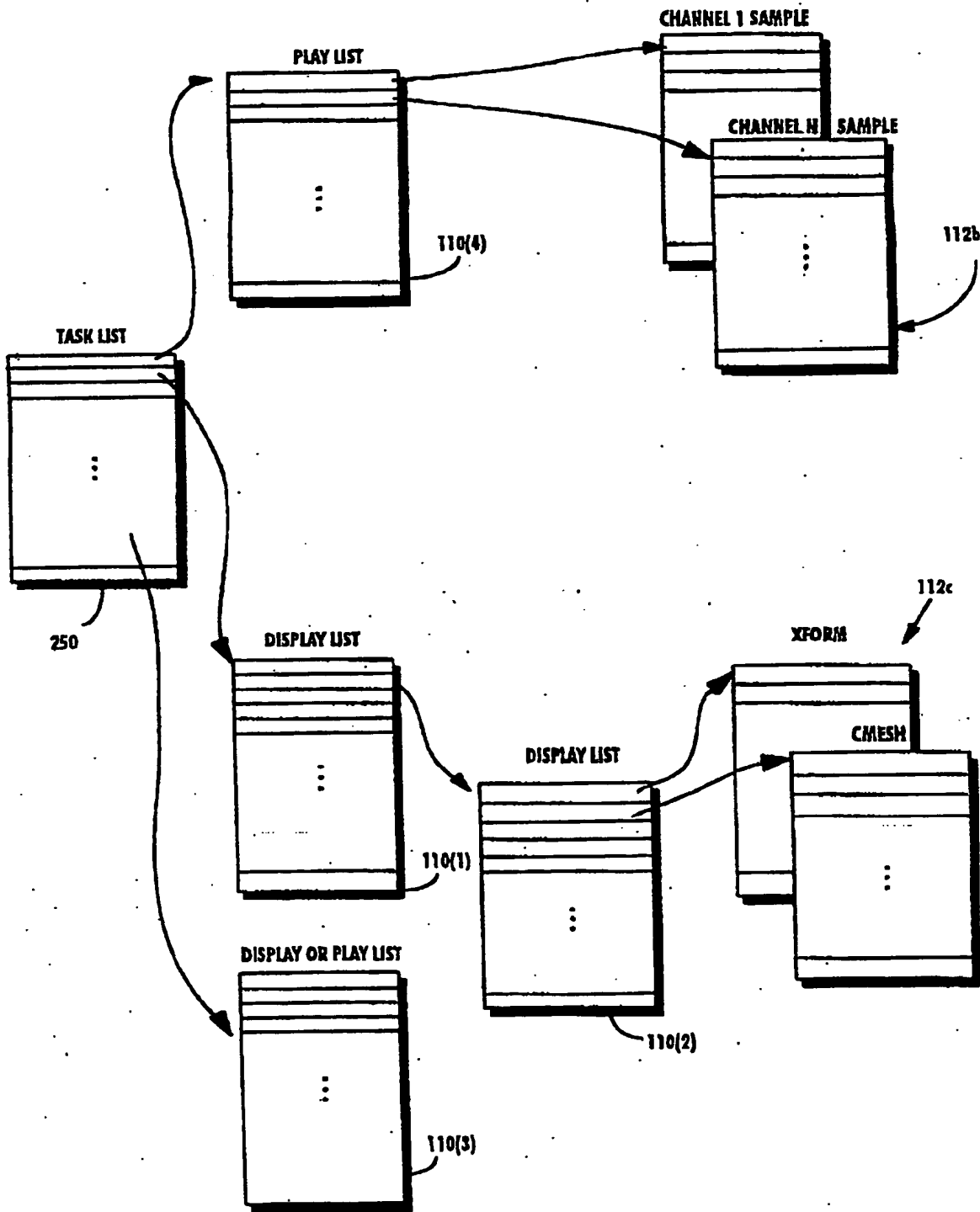
Fig. 8 TASK LIST
